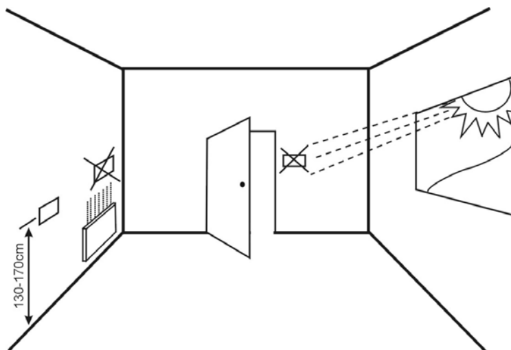
Rys. Prawidłowe umieszczenie regulatora w pomieszczeniu
